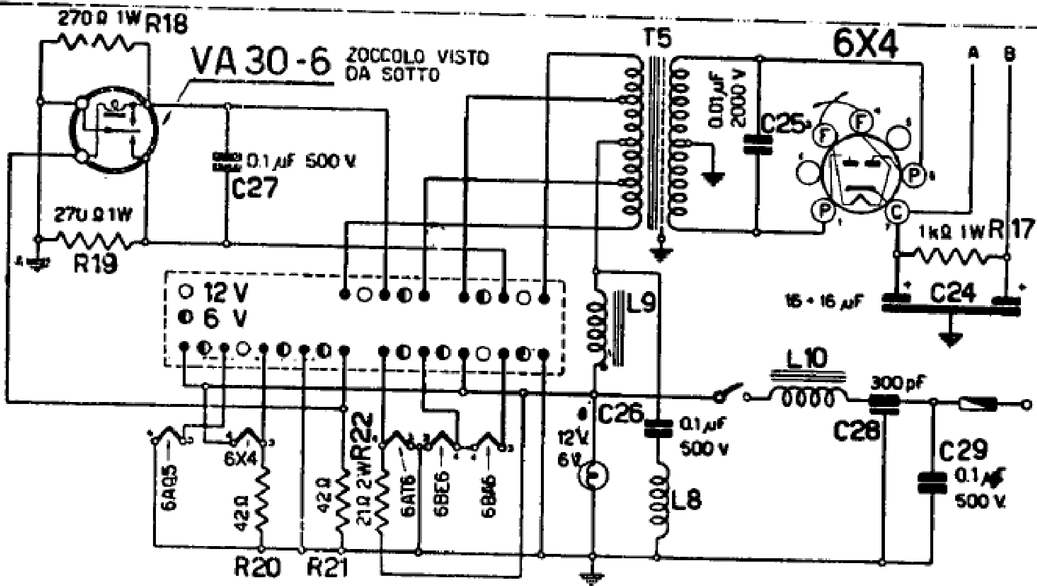
VARIANTE AL CIRCUITO DI ALIMENTAZIONE PER VERSIONE RA 19-E
